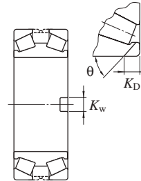
Face key way : B
