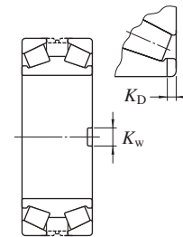
Face key way : A
