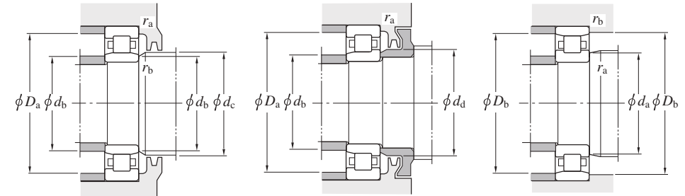
Boundary dimensions (mm) Basic load ratings (kN) Bearing No. 1) De- sign Mounting dimensions (mm) (Refer.) d D B r min. r 1 min. F w E w C r C 0r NU d a min. d b min. d b max. d c min. d d min. D a max. D b max. D b min. r a max. r b max. Mass NU (kg) 120 215 40 2.1 2.1 143.5 191.5 260 318 NU224 1 131 131 141 146 156 204 204 196 2 2 5.65 215 40 2.1 2.1 143.5 195 336 421 NU224R 1 131 131 141 146 156 204 — — 2 2 5.85 215 58 2.1 2.1 143.5 191.5 367 492 NU2224 1 131 131 141 146 156 204 — — 2 2 8.56 215 58 2.1 2.1 143.5 195.5 452 619 NU2224R 1 131 131 141 146 156 204 — — 2 2 8.56 215 76 2.1 2.1 143.5 191.5 477 695 NU3224 1 131 131 141 146 — 204 — — 2 2 11.9 260 55 3 3 154 226 485 551 NU324 1 133 133 151 156 171 247 247 230 2.5 2.5 13.1 260 55 3 3 154 230 528 610 NU324R 1 133 133 151 156 171 247 — — 2.5 2.5 13.4 260 86 3 3 154 226 708 918 NU2324 1 133 133 151 156 171 247 — — 2.5 2.5 23.1 130 180 30 1.5 1.5 142 168 152 243 NU2926 1 138 138 140 145 150 172 172 — 1.5 1.5 2.27 200 33 2 1.1 148 182 171 238 NU1026 1 139 136.5 146 151 — 191 — — 2 1 3.77 230 40 3 3 156 204 282 362 NU226 1 143 143 151 158 168 217 217 208 2.5 2.5 6.49 230 40 3 3 153.5 209 364 453 NU226R 1 143 143 151 158 168 217 — — 2.5 2.5 6.60 230 64 3 3 156 204 395 560 NU2226 1 143 143 151 158 168 217 — — 2.5 2.5 11.2 230 64 3 3 153.5 209.5 530 737 NU2226R 1 143 143 151 158 168 217 — — 2.5 2.5 11.2 230 80 3 3 156 204 550 857 NU3226 1 143 143 151 158 — 217 — — 2.5 2.5 14.1 280 58 4 4 167 243 564 667 NU326 1 146 146 164 169 184 264 264 247 3 3 16.4 280 58 4 4 167 247 616 736 NU326R 1 146 146 164 169 184 264 — — 3 3 16.7 280 93 4 4 167 243 838 1 130 NU2326 1 146 146 164 169 184 264 — — 3 3 29.1 280 93 4 4 167 247 920 1 230 NU2326R 1 146 146 164 169 186 264 — — 3 3 29.1 280 112 4 4 167 243 936 1 290 NU3326 1 146 146 164 169 — 264 — — 3 3 34.6 140 190 30 1.5 1.5 152 178 165 275 NU2928 1 148 148 151 155 161 182 182 180 1.5 1.5 2
